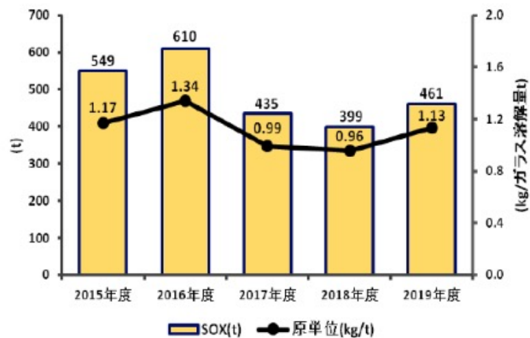
SO x 排出量と原単位
