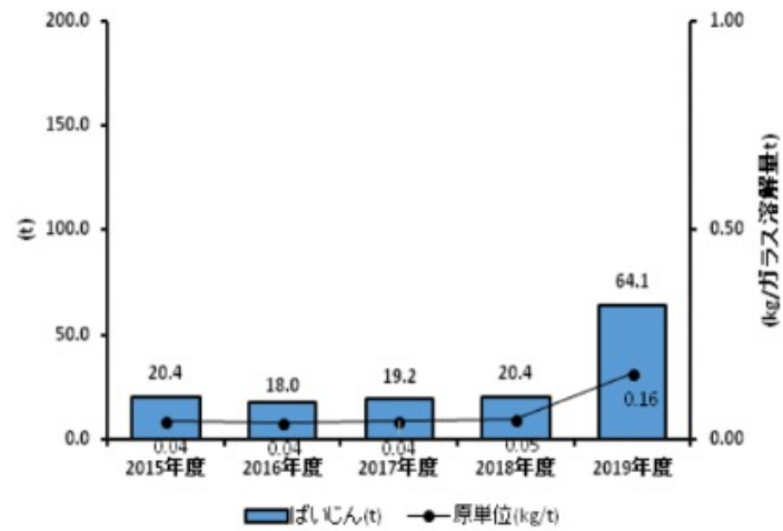
ばいじん排出量と原単位
