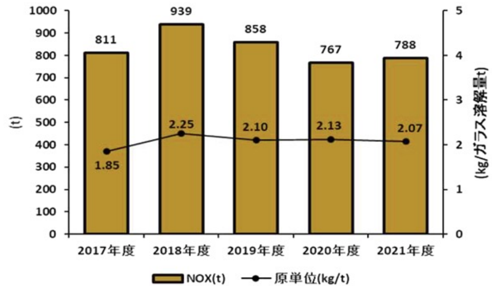
NO x 排出量と原単位
