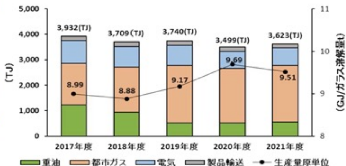
エネルギー使用量と原単位
